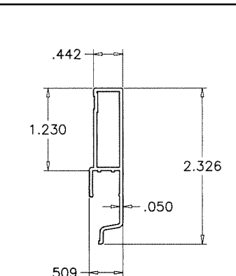
(2A) SILL RISER (3 TRACK)
