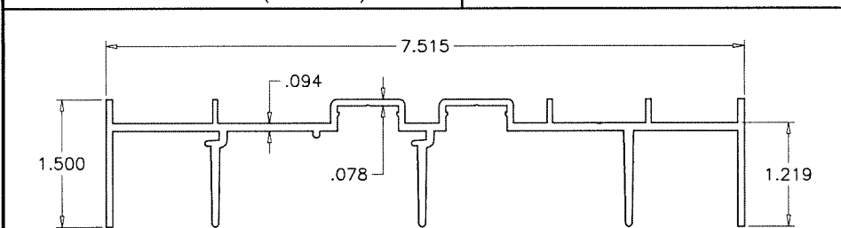
(3.1) FRAME JAMB (3 TRACK)
